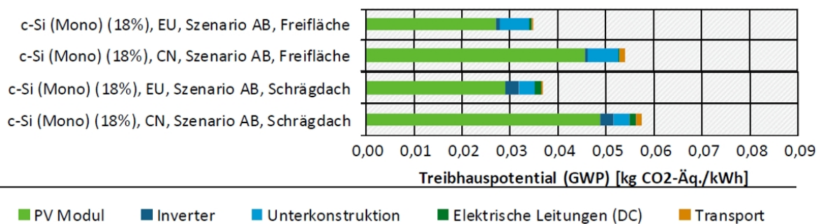
Abbildung 42: Treibhauspotential der Stromerzeugung mit mono c-Si PV für Dach- und Freiflächenanlagen [UBA7].
